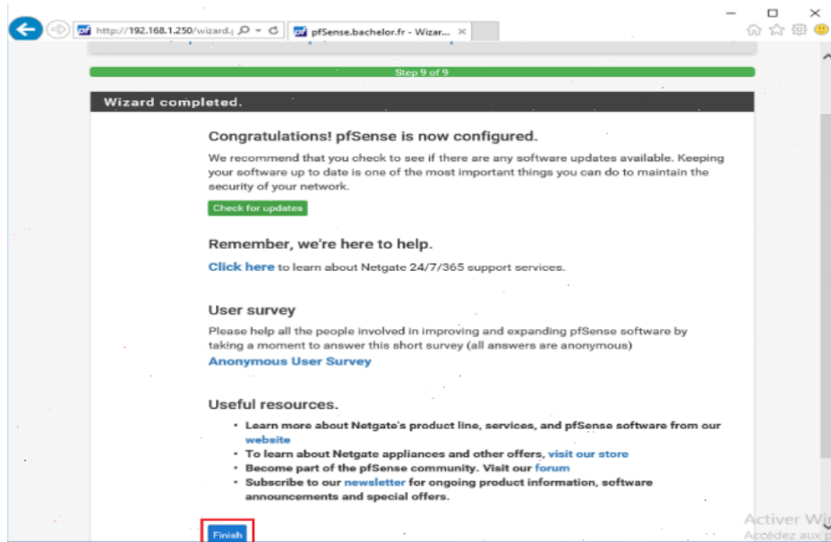
Assistant de configuration PfSense – étape 10
