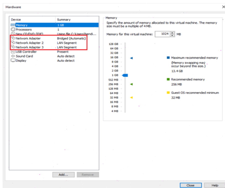
Étape d'installation PfSense – écran 7
